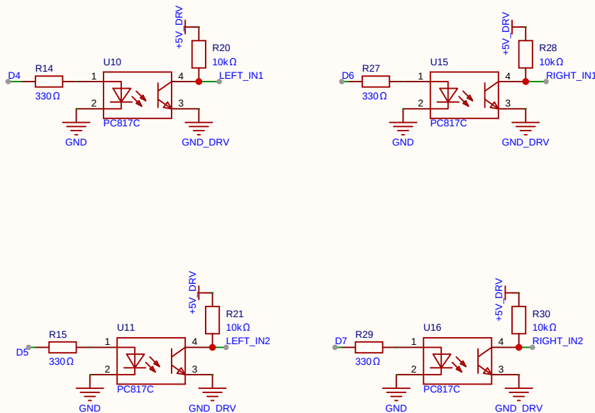
PC817连接
